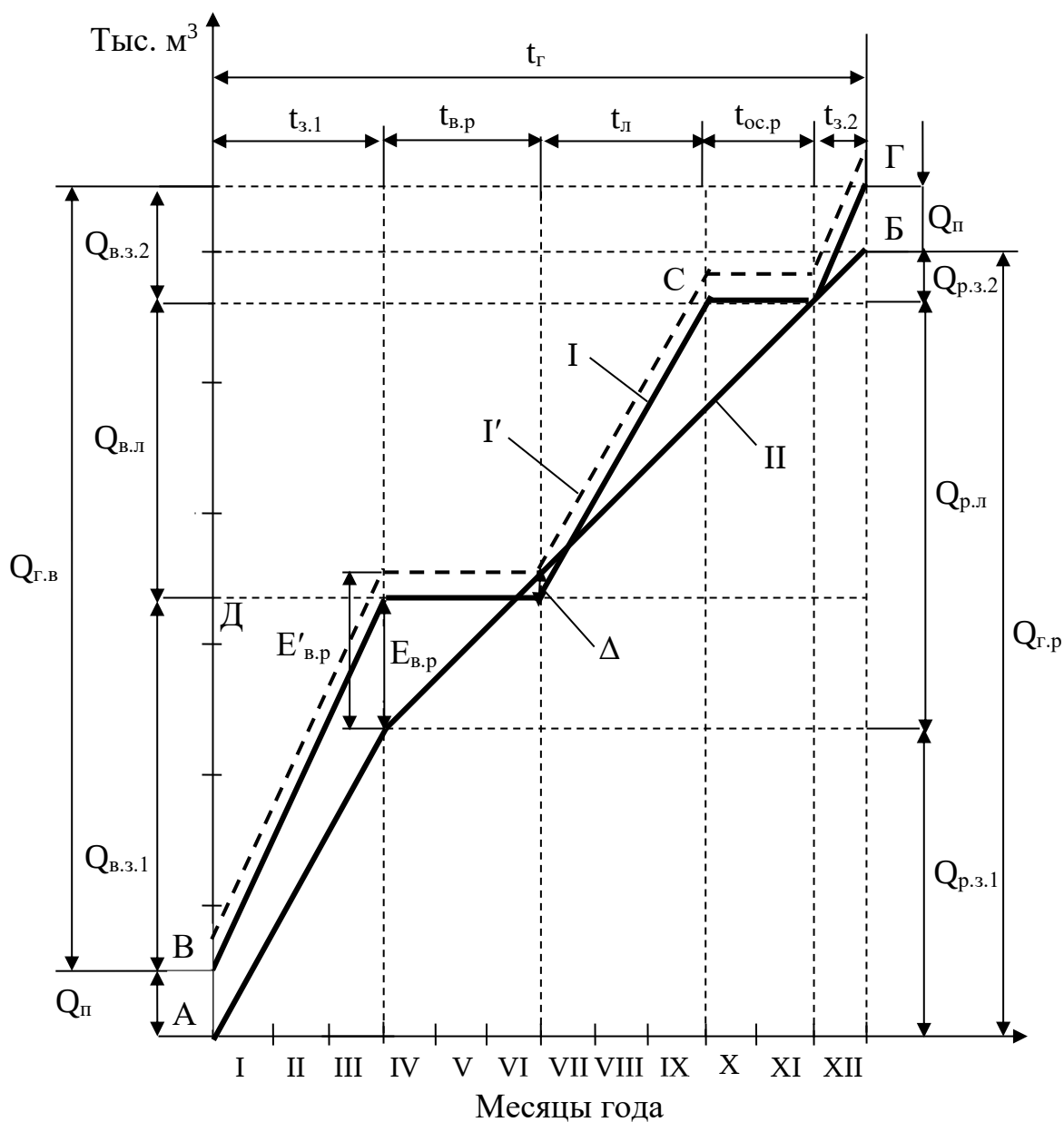
Рис. 1.2. Интегральные графики режима работы нижнего лесопромышленного склада при неравномерной раскряжевке хлыстов: I, I' – графики поступления хлыстов на склад; II – график раскряжевки хлыстов
