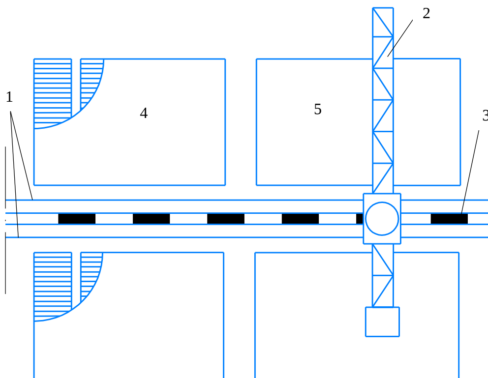
Рис. П4.4.1. Схема склада круглых лесоматериалов на базе башенного крана КБ-572: 1 – подкрановые пути; 2 – кран КБ-572; 3 – тупик РЖД; 4 – штабеля круглых лесоматериалов на отгрузку; 5 – штабеля круглых лесоматериалов на переработку
