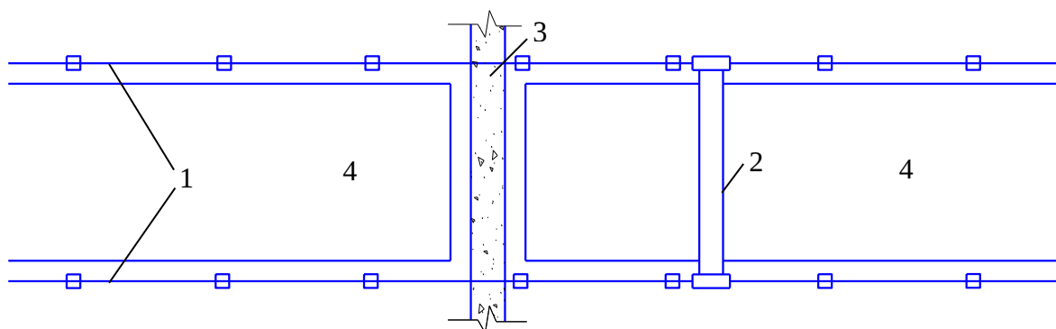
Рис. П1.2.2. Схема склада хлыстов на базе мостового крана: 1 – подкрановые пути; 2 – кран мостовой; 3 – автомобильная дорога; 4 – штабель хлыстов
