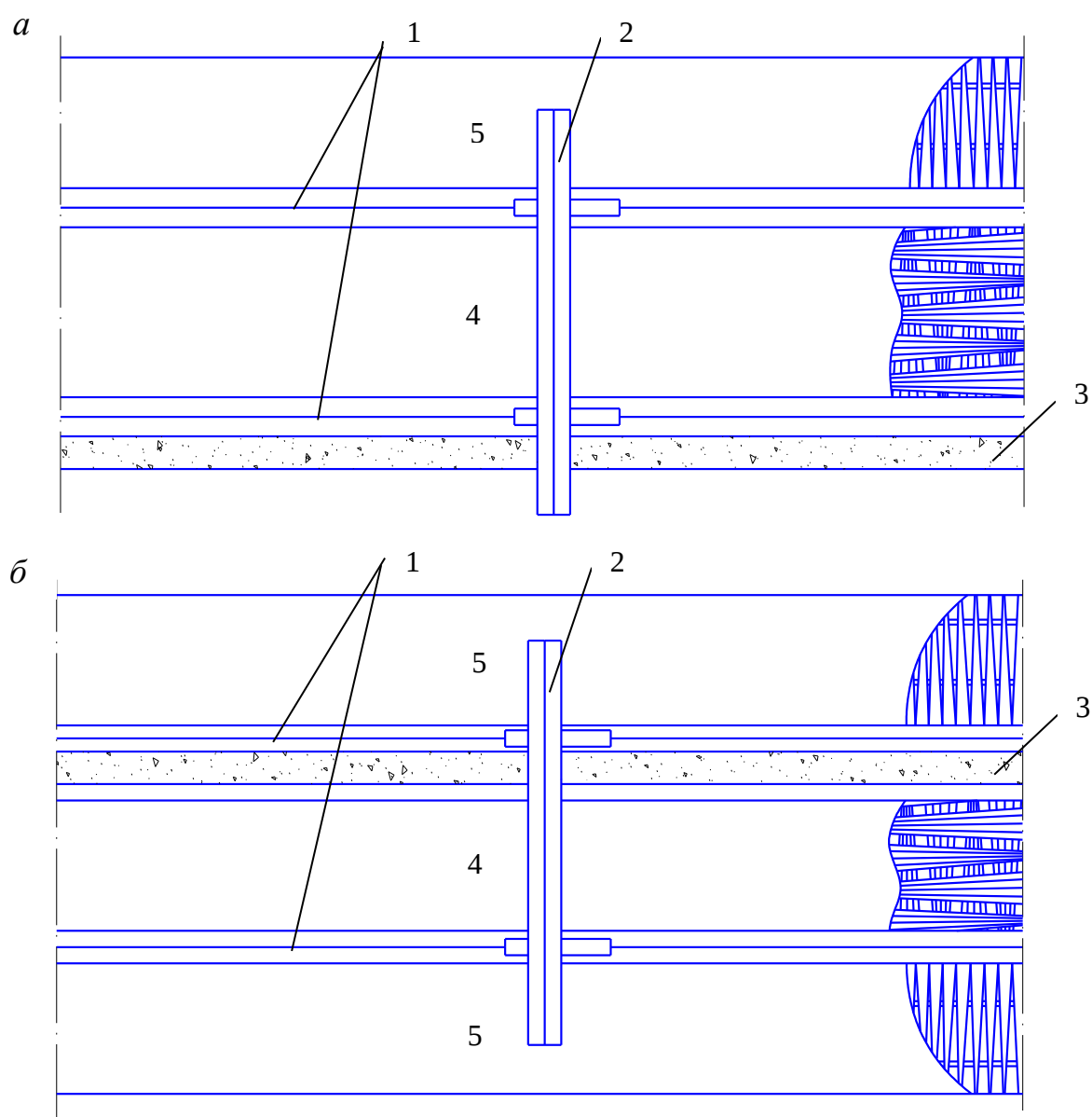
Рис. П1.2.1. Схема склада хлыстов на базе консольно-козлового крана ККЛ-32: а – с расположением автомобильной лесовозной дороги под консолью крана; б – с расположением автомобильной лесовозной дороги в пролете крана (1 – подкрановые пути; 2 – кран консольно-козловой; 3 – автомобильная дорога; 4 – штабель хлыстов в пролете крана; 5 – штабель хлыстов под консолью крана)
