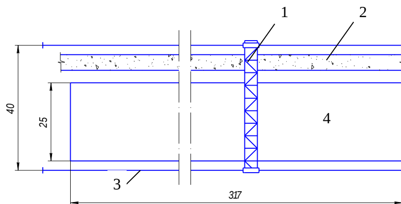
Рис. П1.3.1. Схема склада хлыстов на базе козлового крана ЛТ-62: 1 – кран ЛТ-62; 2 – автомобильная дорога; 3 – подкрановые пути; 4 – штабель хлыстов
