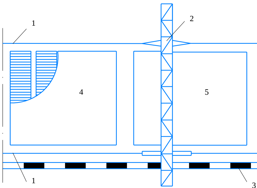
Рис. П4.4.2. Схема склада круглых лесоматериалов на базе консольно-козлового крана ККС-10: 1 – подкрановые пути; 2 – кран ККС-10; 3 – тупик РЖД; 4 – штабеля круглых лесоматериалов на отгрузку; 5 – штабеля круглых лесоматериалов на переработку
