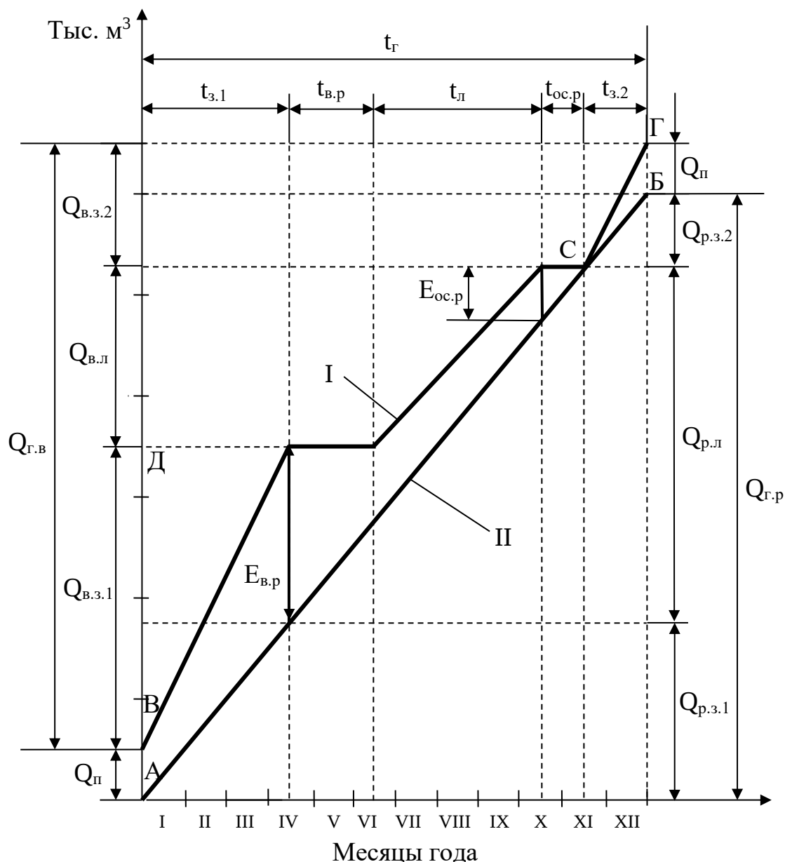
Рис. 1.1. Интегральные графики режима работы нижнего лесопромышленного склада при равномерной раскряжевке хлыстов: I – график поступления хлыстов на склад; II – график раскряжевки хлыстов
