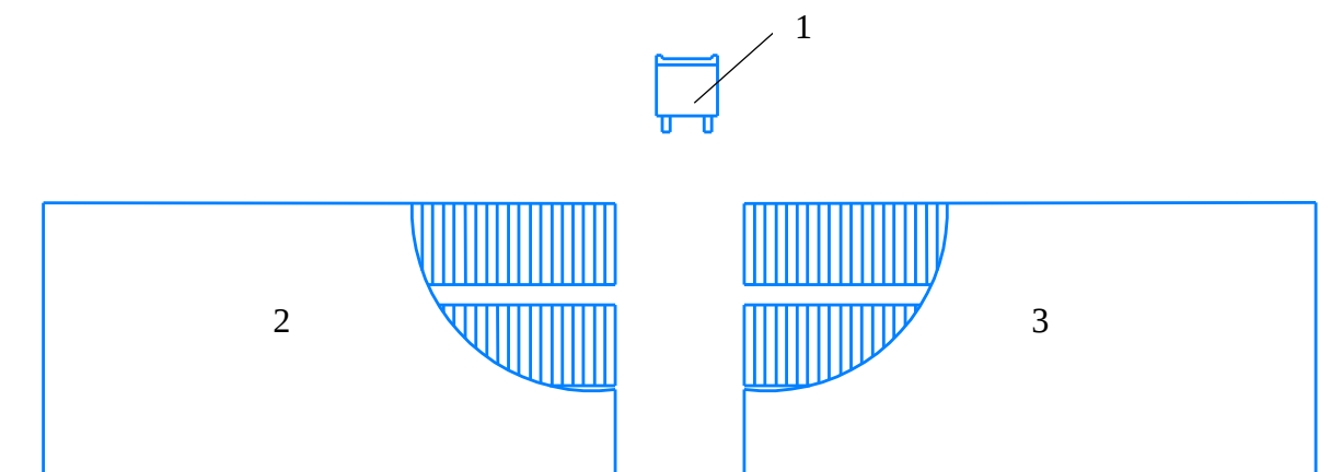
Рис. П4.4.3. Схема склада круглых лесоматериалов на базе колесного погрузчика: 1 – колесный погрузчик; 2 – штабеля круглых лесоматериалов на отгрузку; 3 – штабеля круглых лесоматериалов на переработку
